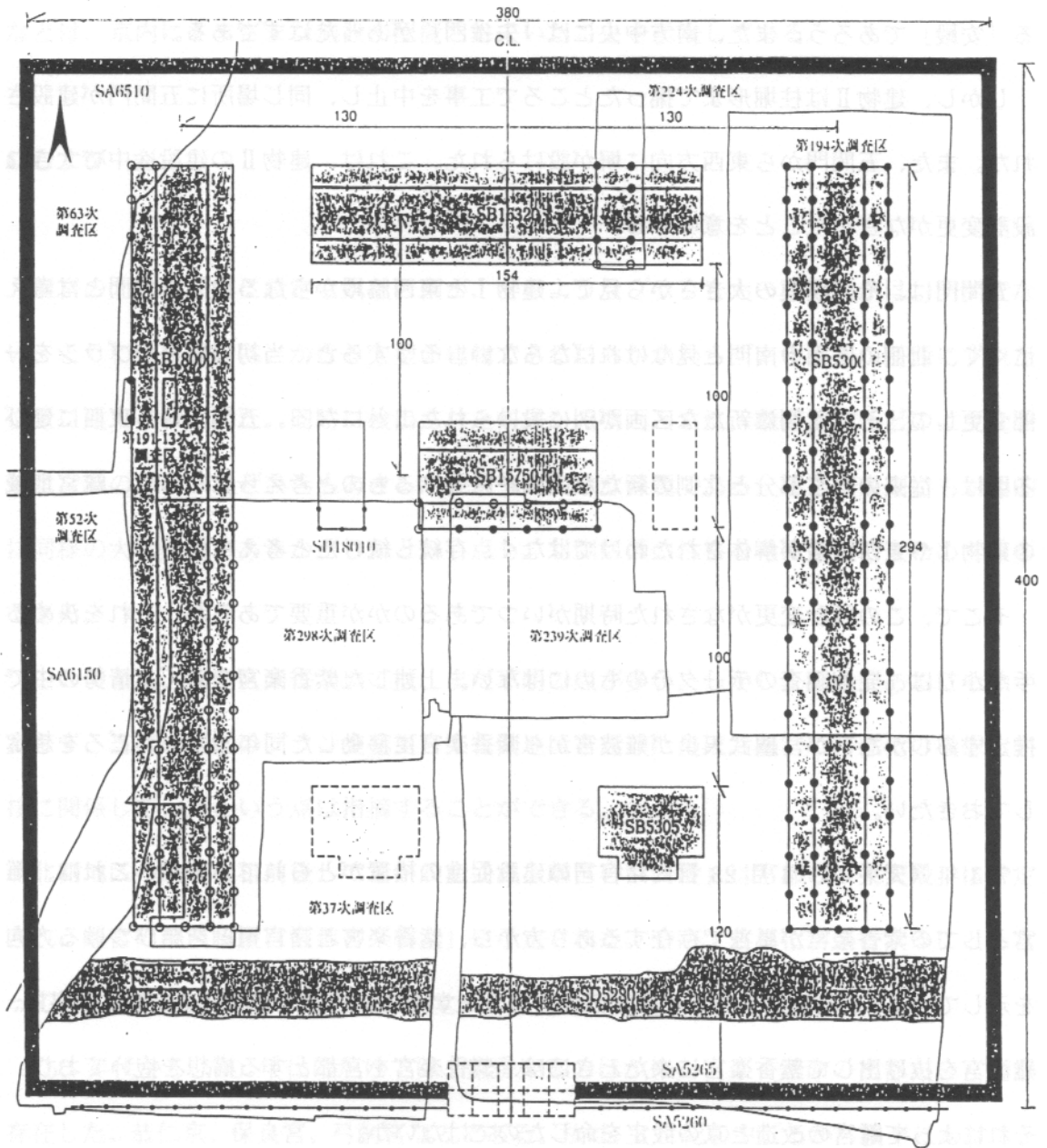
图 11 馬寮東方東区建物配置図 (单位：尺 1:800)
